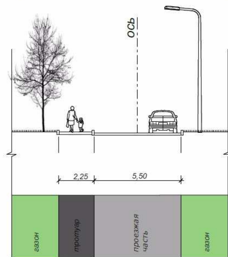
Поперечный профиль местного проезда
