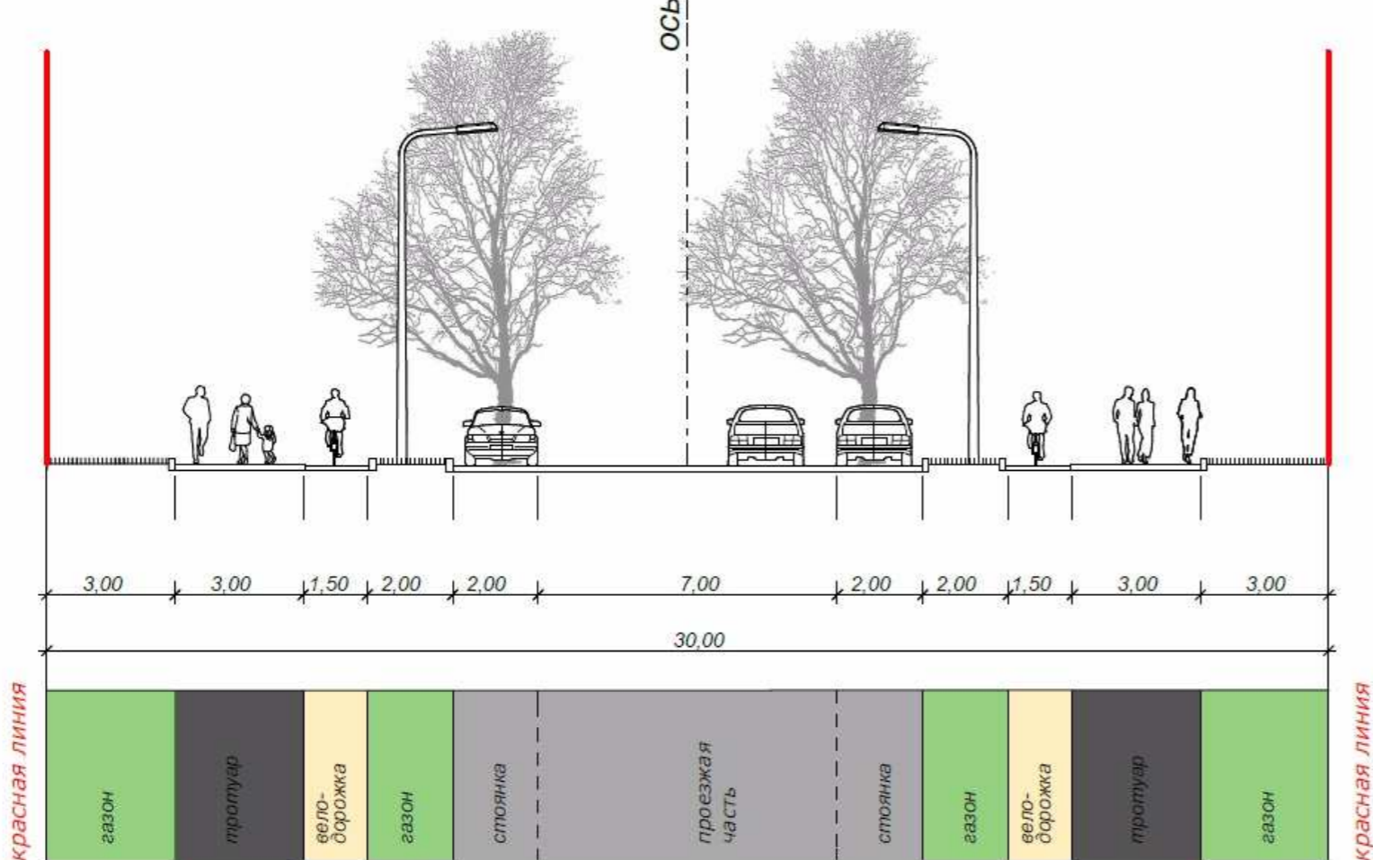
Поперечный профиль транспортно-пешеходной улицы в жилой застройке
