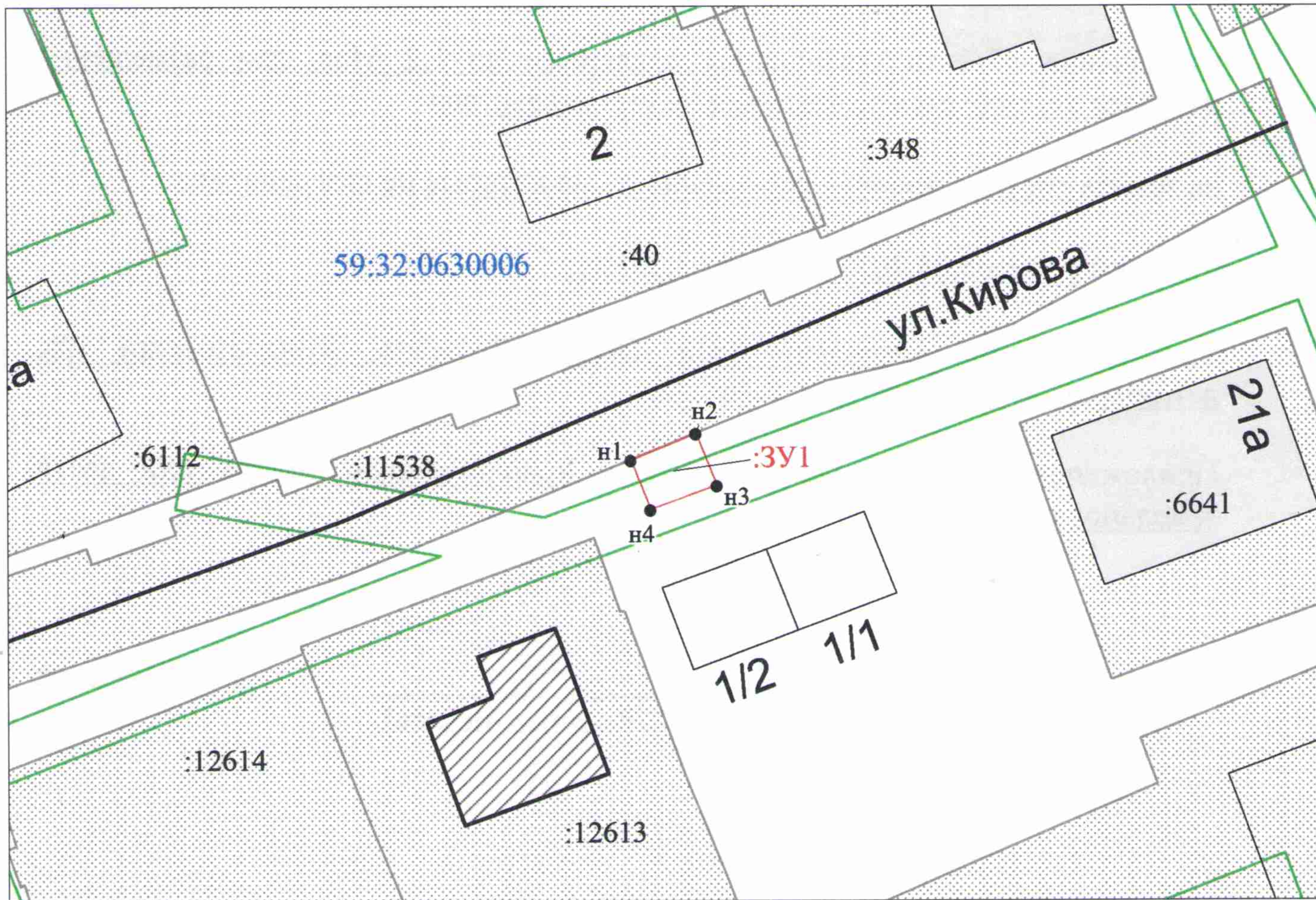
Масштаб 1:500
