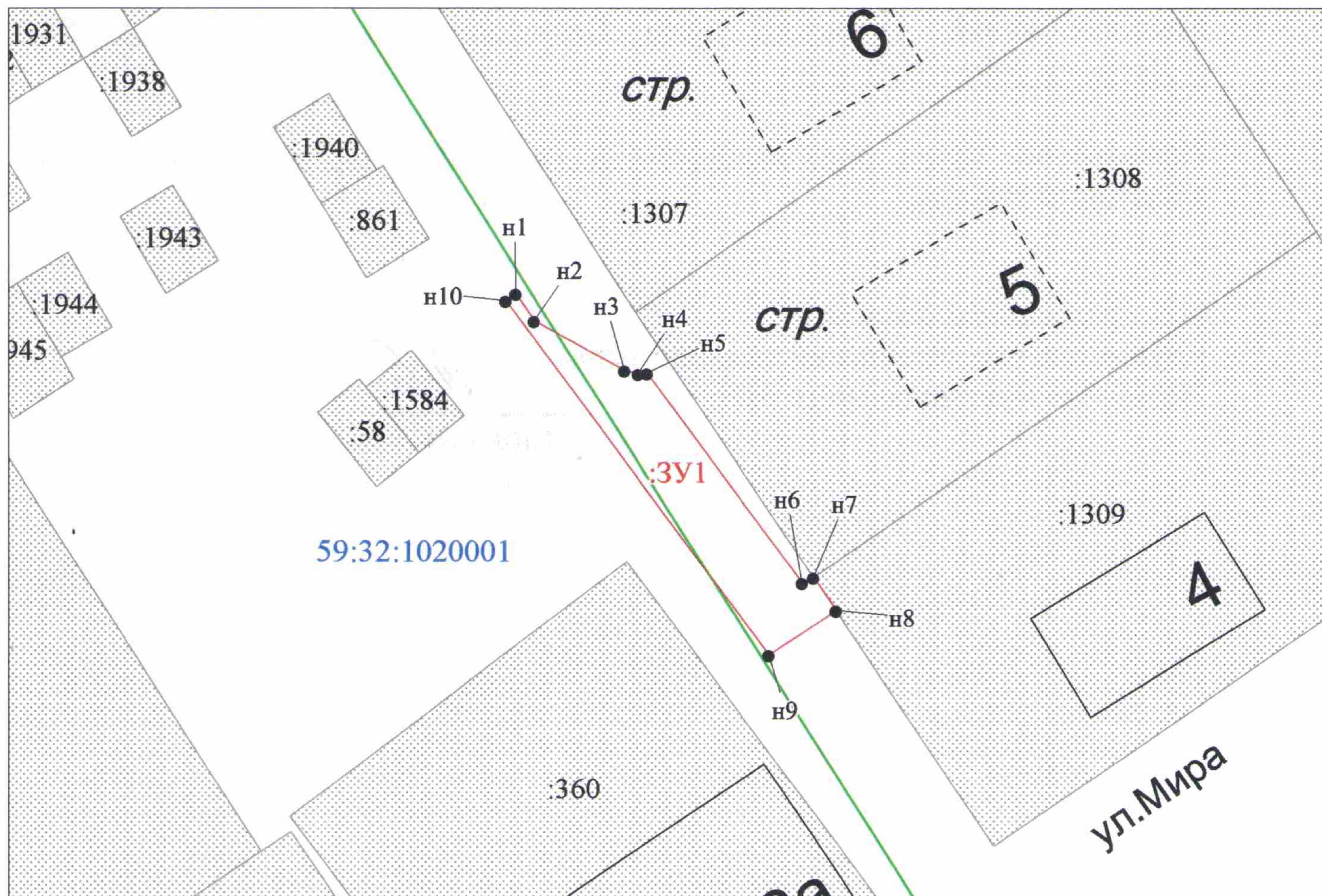
Масштаб 1:500
