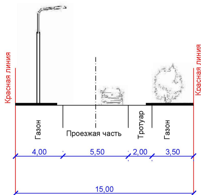
Поперечный профиль местного проезда
